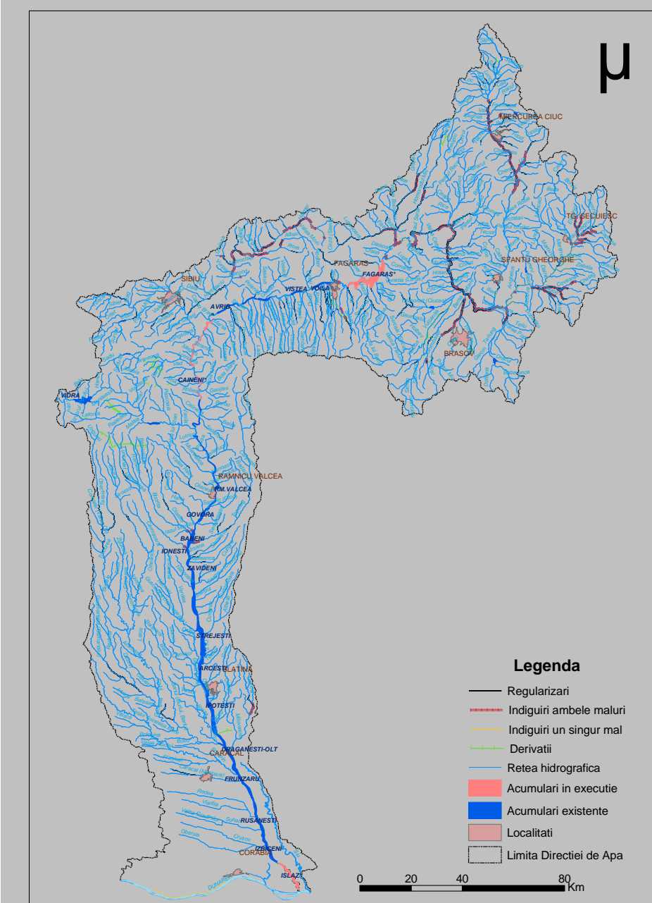
Fig. 3.11 Lucrari hidrotehnice in bazinul hidrografic Olt
